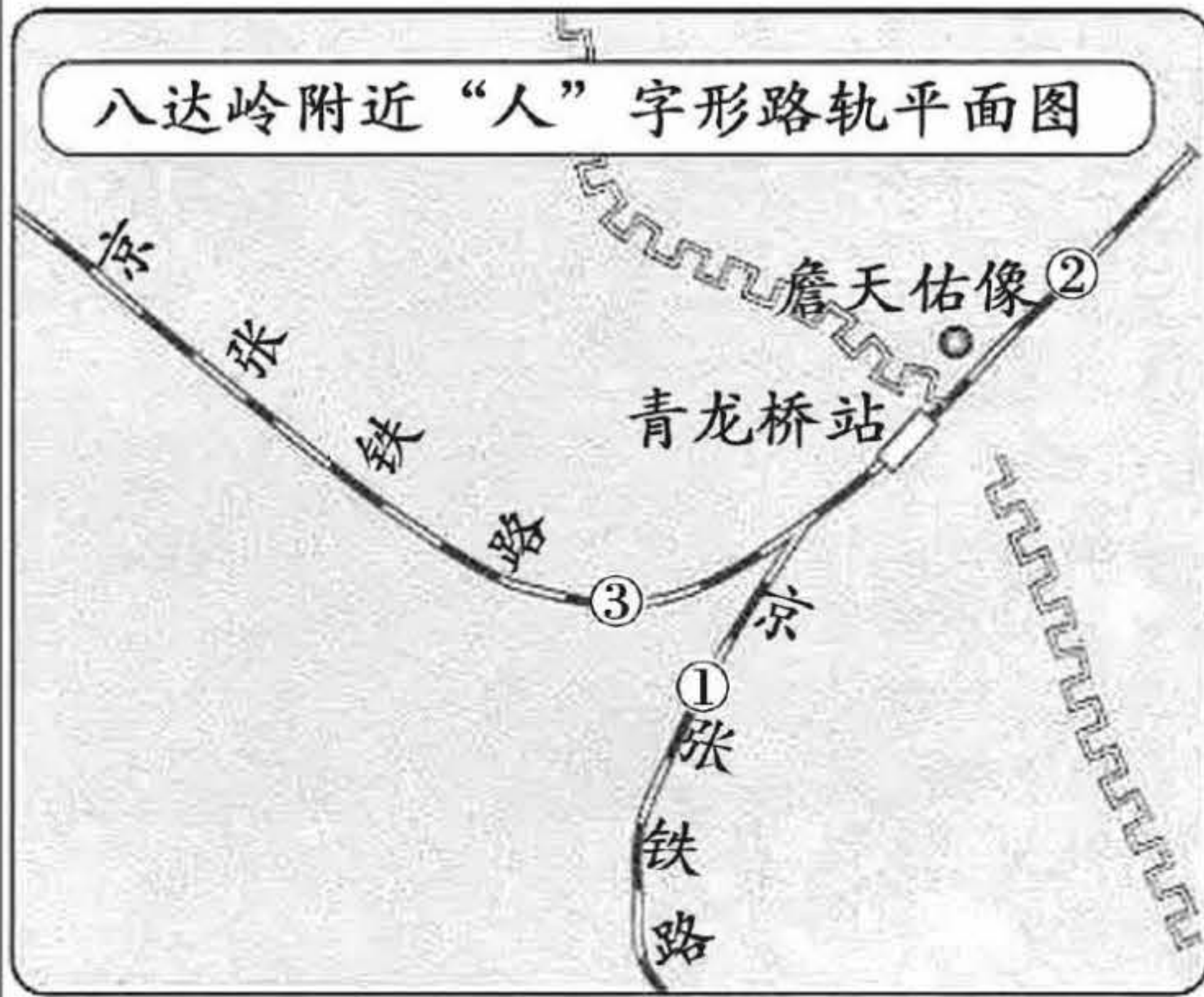
⑦八达岭附近“人”字形路轨平面图
